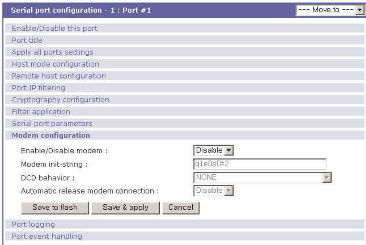
그림 4-16 모뎀 구성
