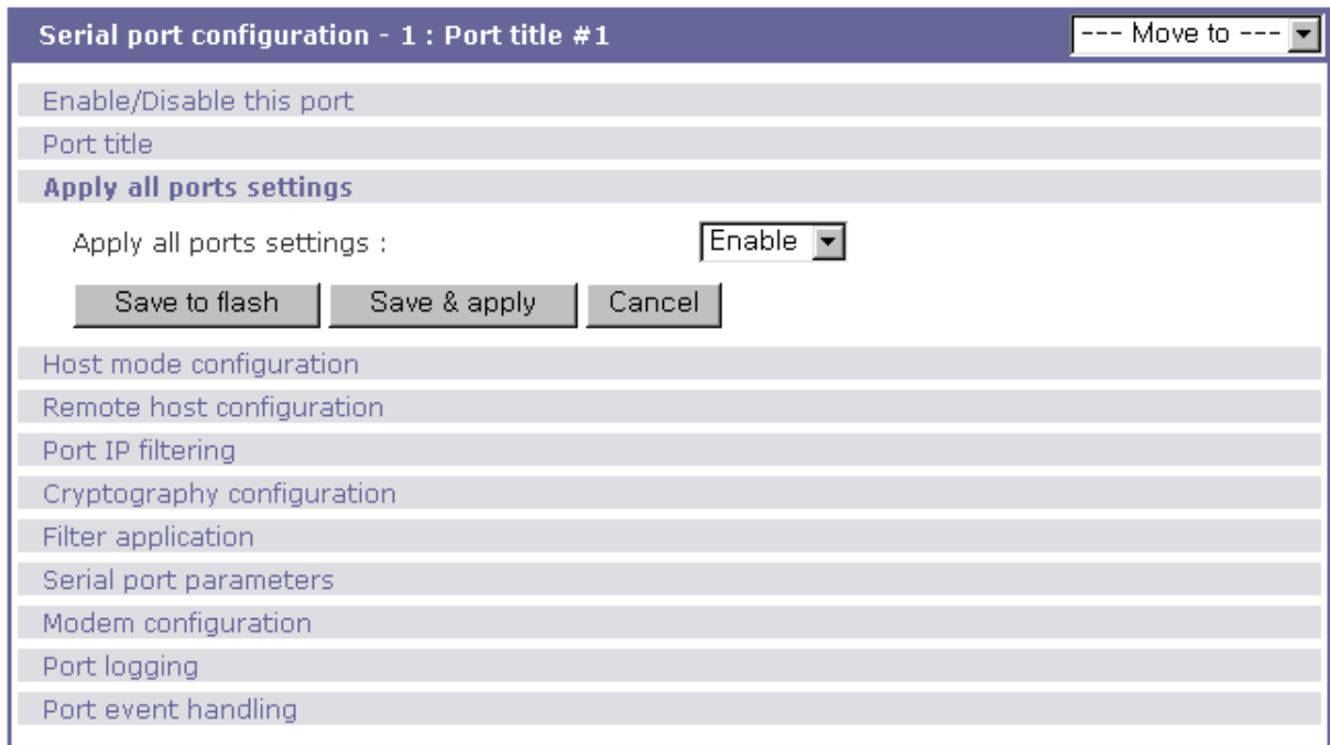
그림 4-4 Apply all port setting configuration.
