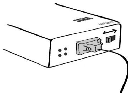
그림 2-13 PS110에 시스템 콘솔 케이블을 연결하기
