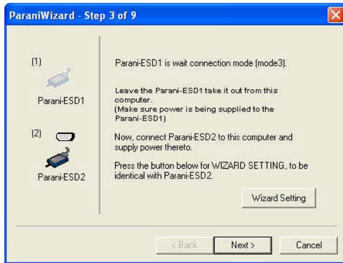
그림 3-12 ParaniWizard Step 3
