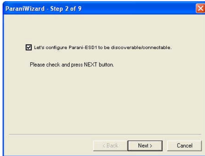
그림 3-11 ParaniWizard Step 2
