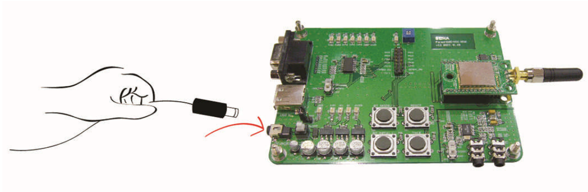
그림 Error! Style not defined. -4 개발 보드에 전원 연결
