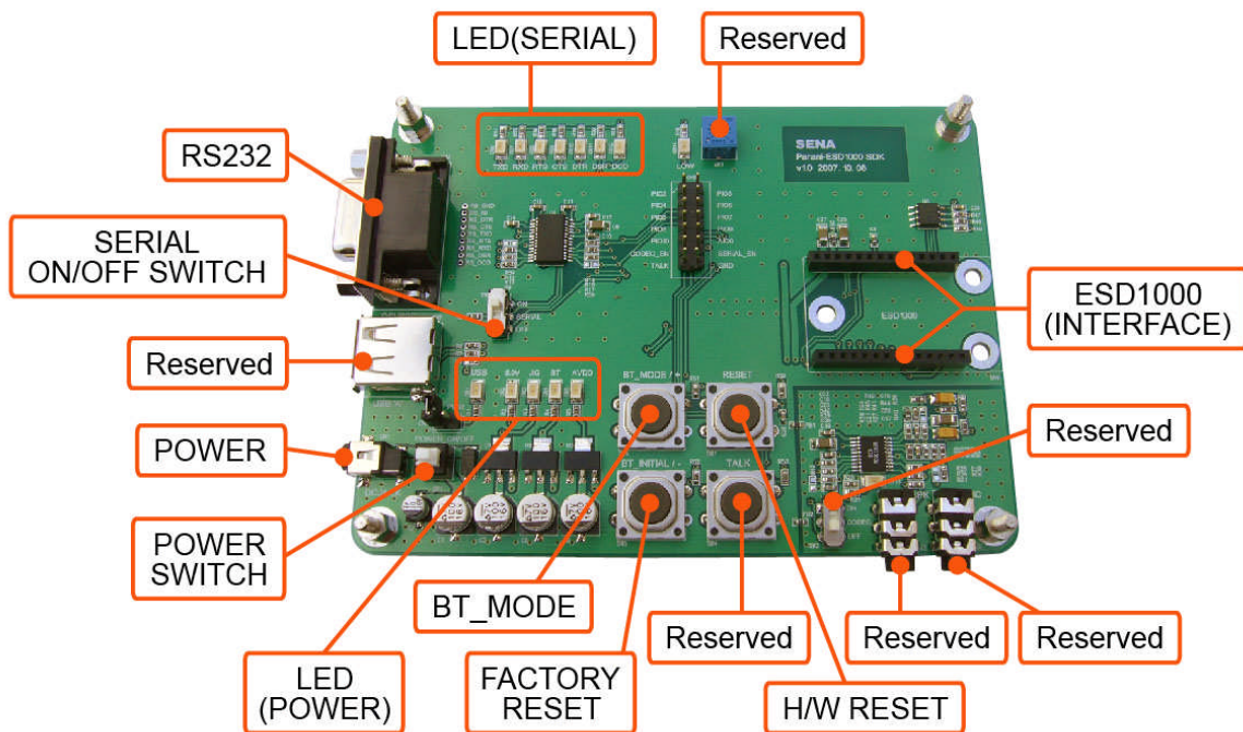
그림 Error! Style not defined.-1 개발 보드 패널 배치
