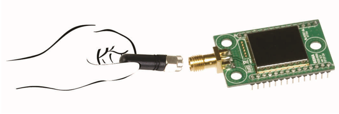
그림 2-2 안테나를 Parani-ESD 모듈에 연결
