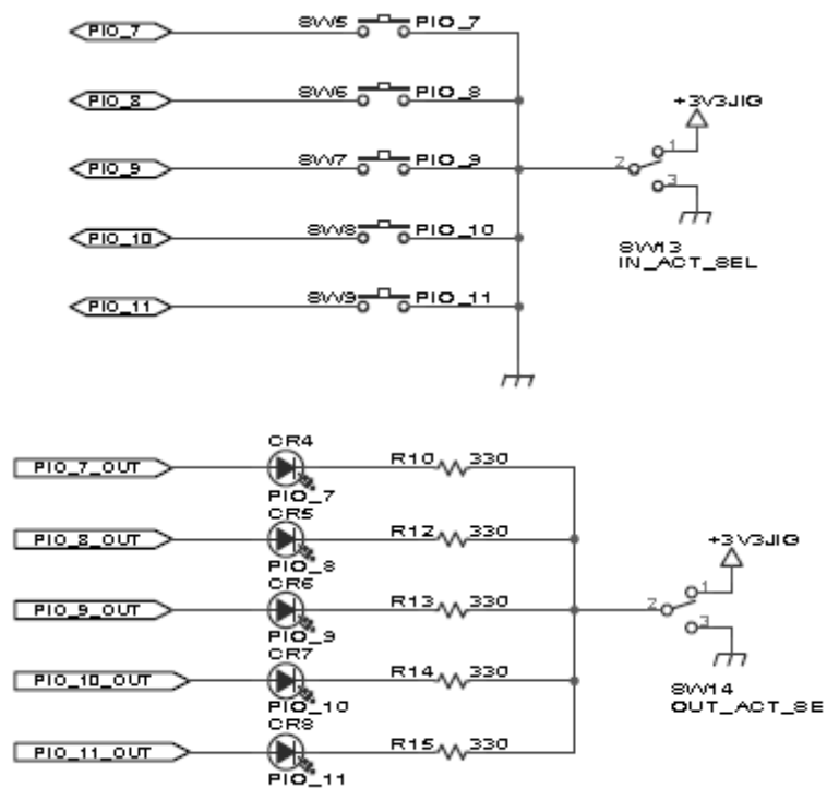
[GPIO 인터페이스]
