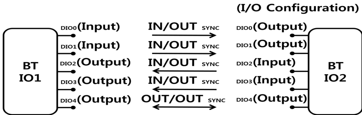
그림 5-2 DIO의 동기화
