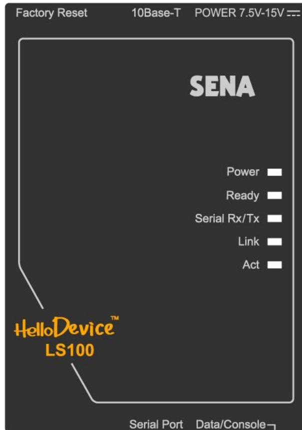
그림 2-1 LS100의 패널 배치
