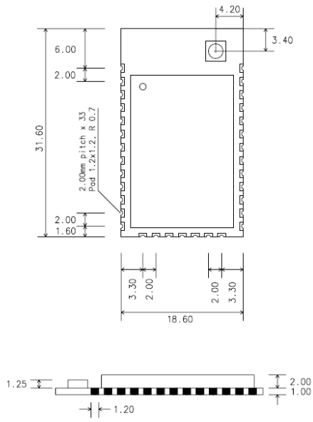
그림 1-6 ProBee-ZE20SSU 치수도
