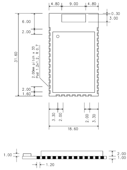
그림 1-7 ProBee-ZE20SSC 치수도
