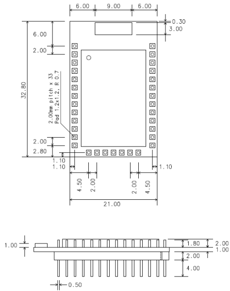
그림 1-5 ProBee-ZE20SDC 치수도
