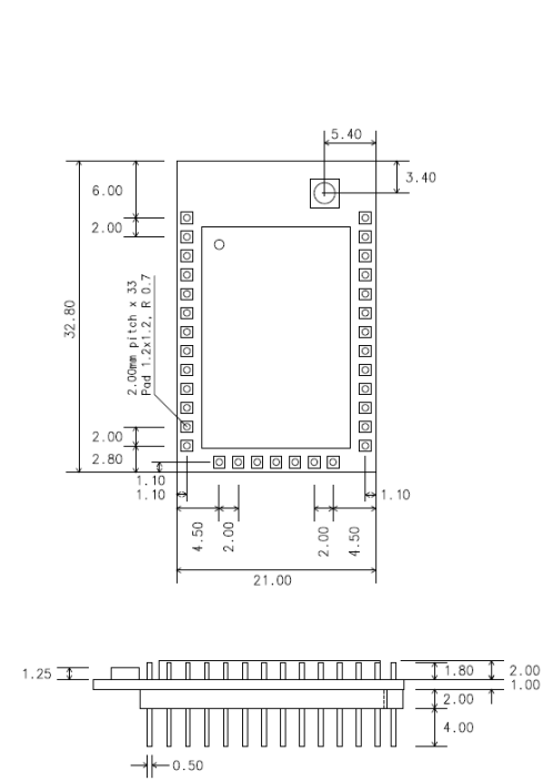
그림 1-3 ProBee-ZE20SDU 치수도
