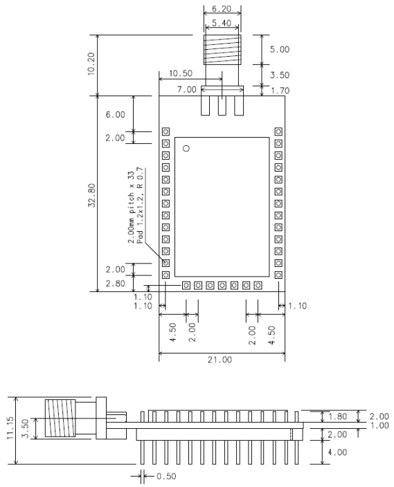
그림 1-4 ProBee-ZE20SDS 치수도
