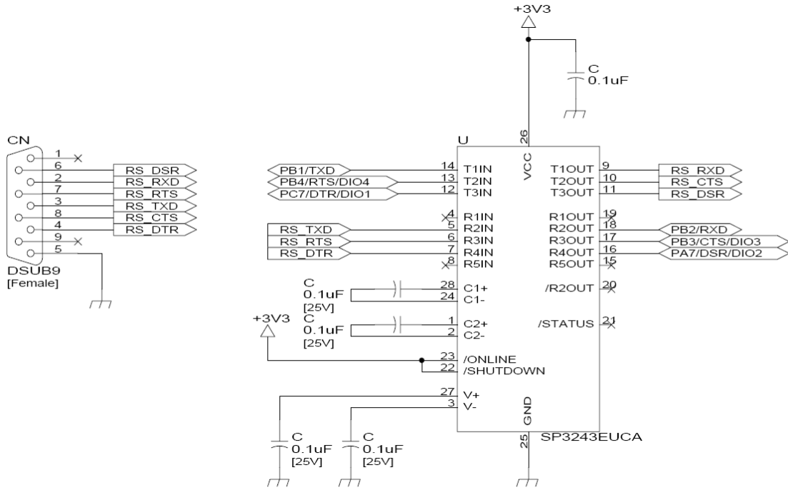
그림 5-3 RS232 시리얼
