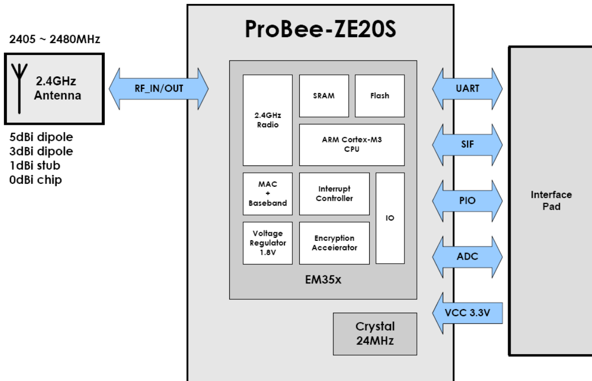
그림 1-1 블록 다이어그램
