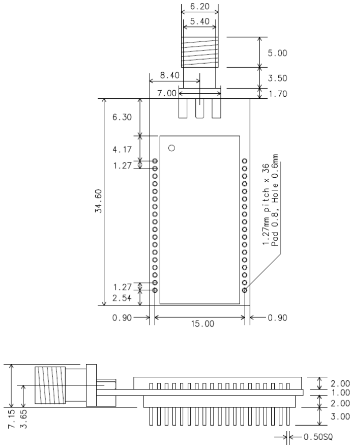
그림 1-7 BCD110DS 치수
