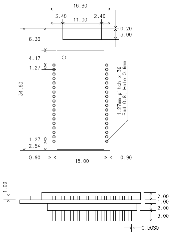
그림 1-6 BCD110DC 치수
