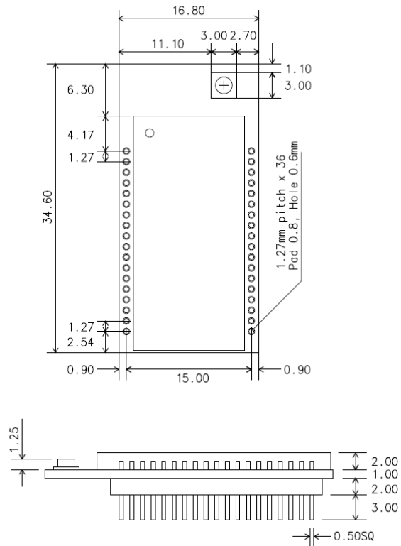
그림 1-4 BCD110DU 치수
