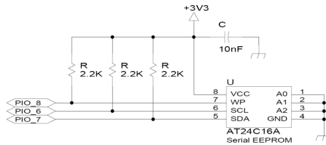
그림 5-6 I2C 인터페이스
