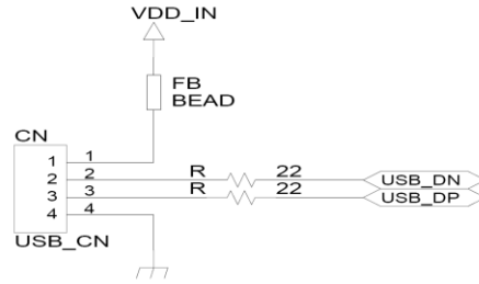
그림 5-5 USB 인터페이스
