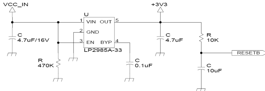
[리셋 인터페이스]
