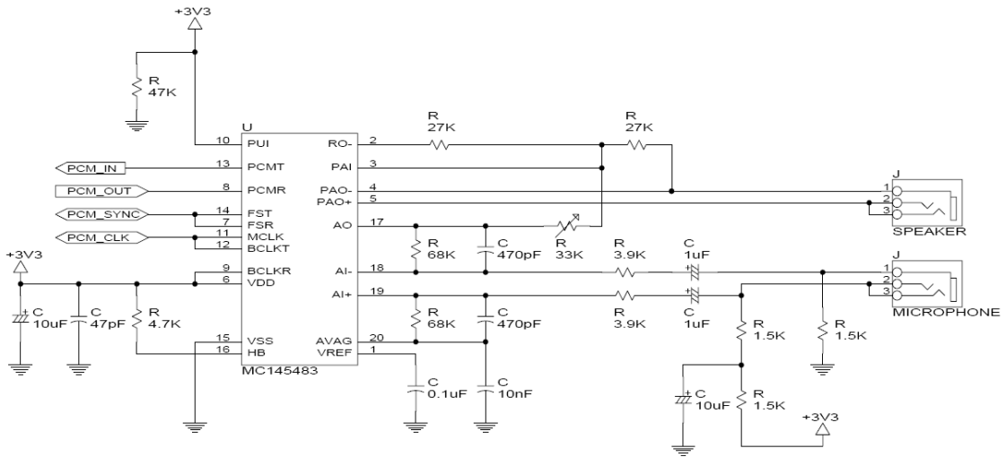
[PCM 인터페이스]
