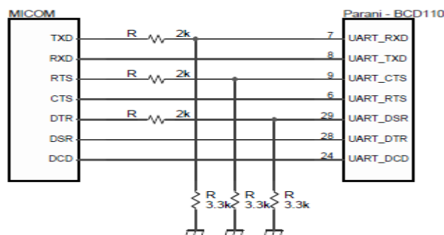
그림 5-4 MICOM UART 인터페이스
