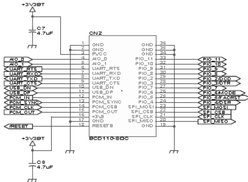
그림 5-1 BT 모듈 인터페이스
