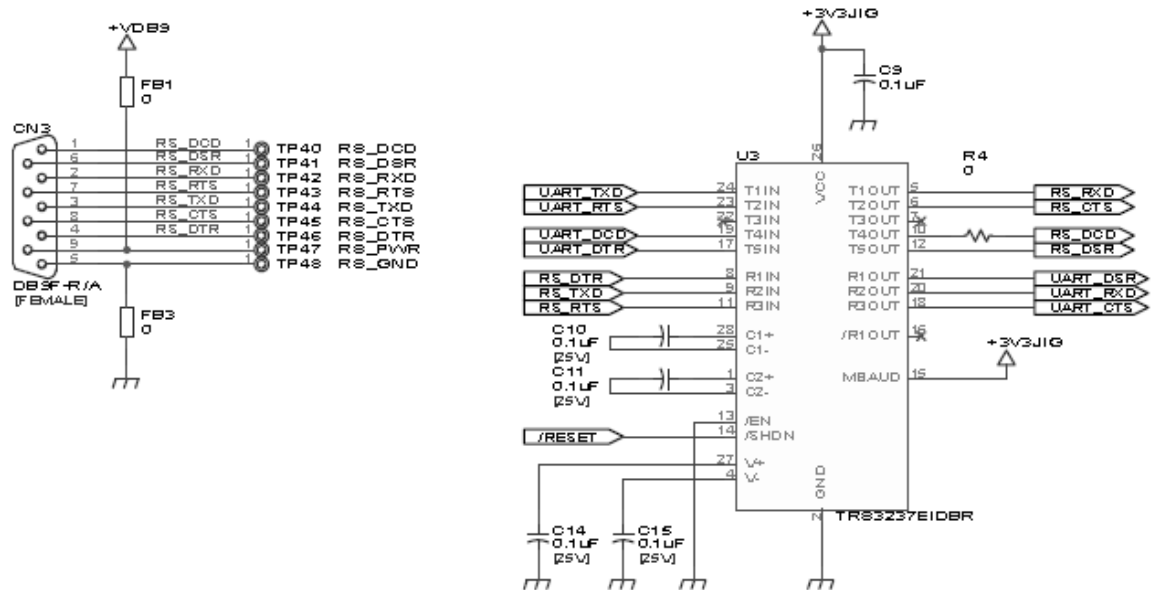
그림 5-3 RS232 시리얼 인터페이스
