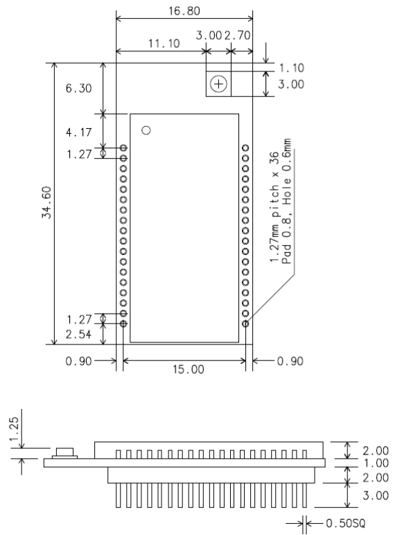
그림 1-4 BCD110DU 치수
