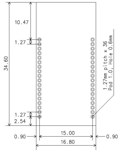
[DIP 타입]
