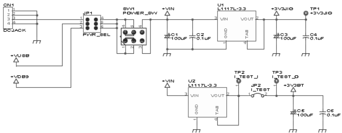
그림 5-2 전원 및 리셋 인터페이스
